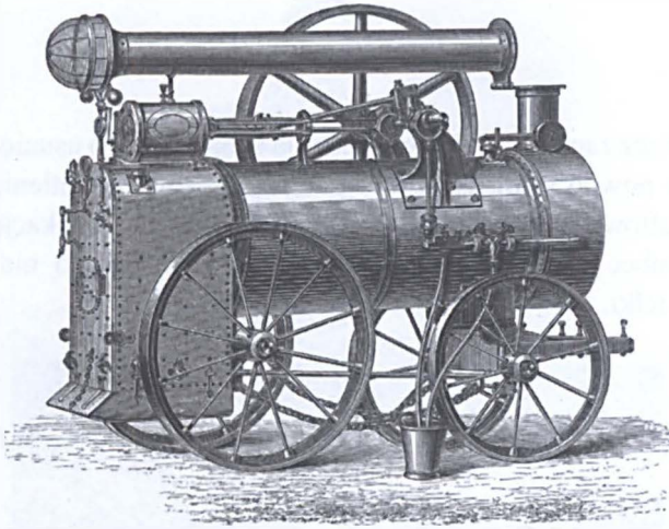
Fig. 1. Lokomobile von Garrett.
